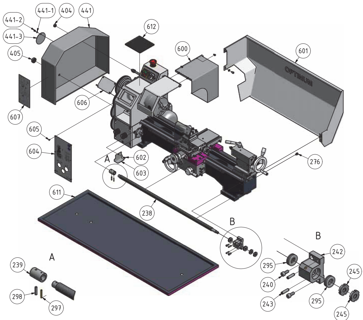
Abb. 1-5: Maschinenbett - Machine bed TU 2506
